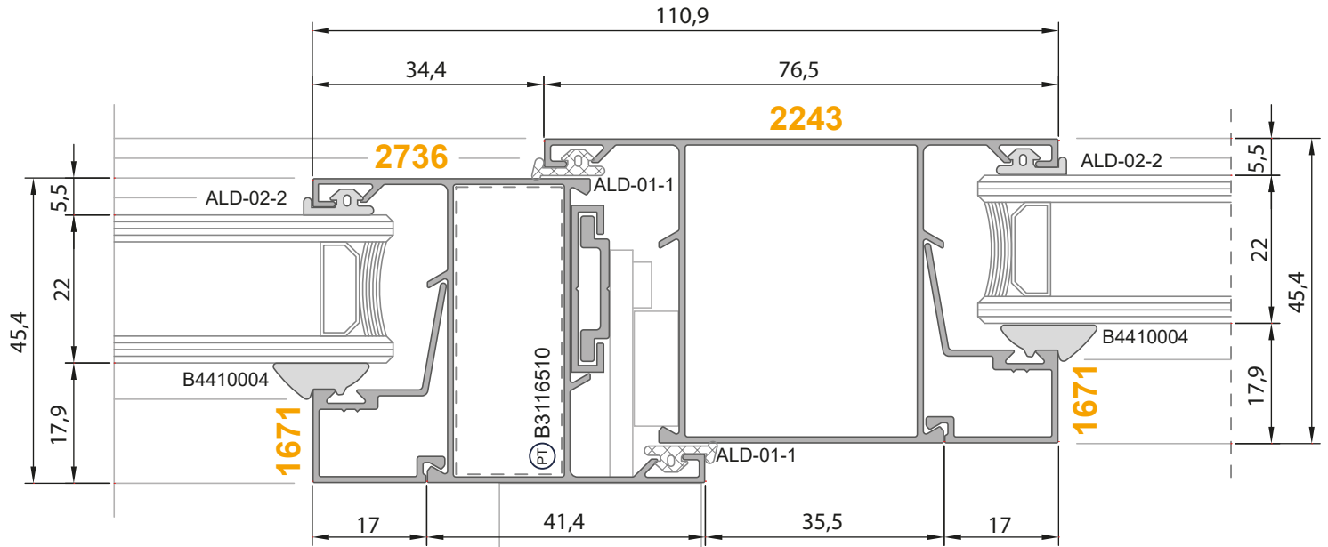
4-4 Detay
