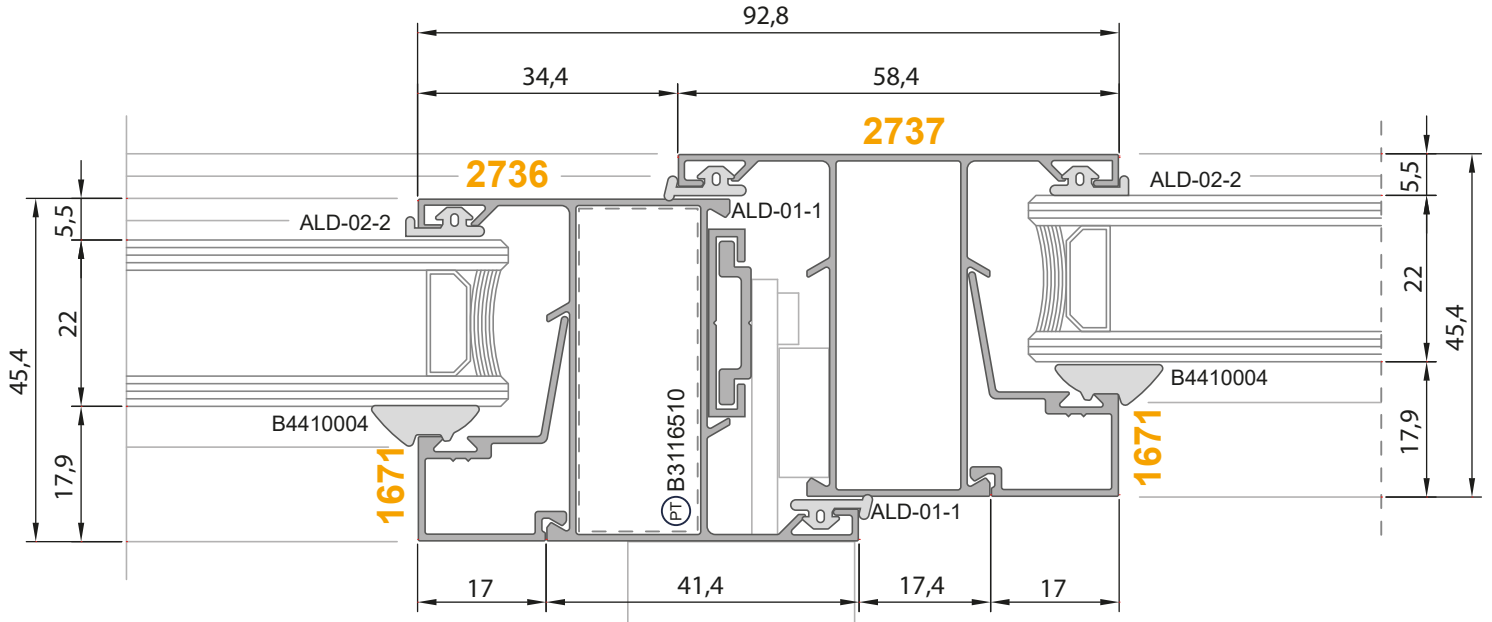
4-4 Detay
