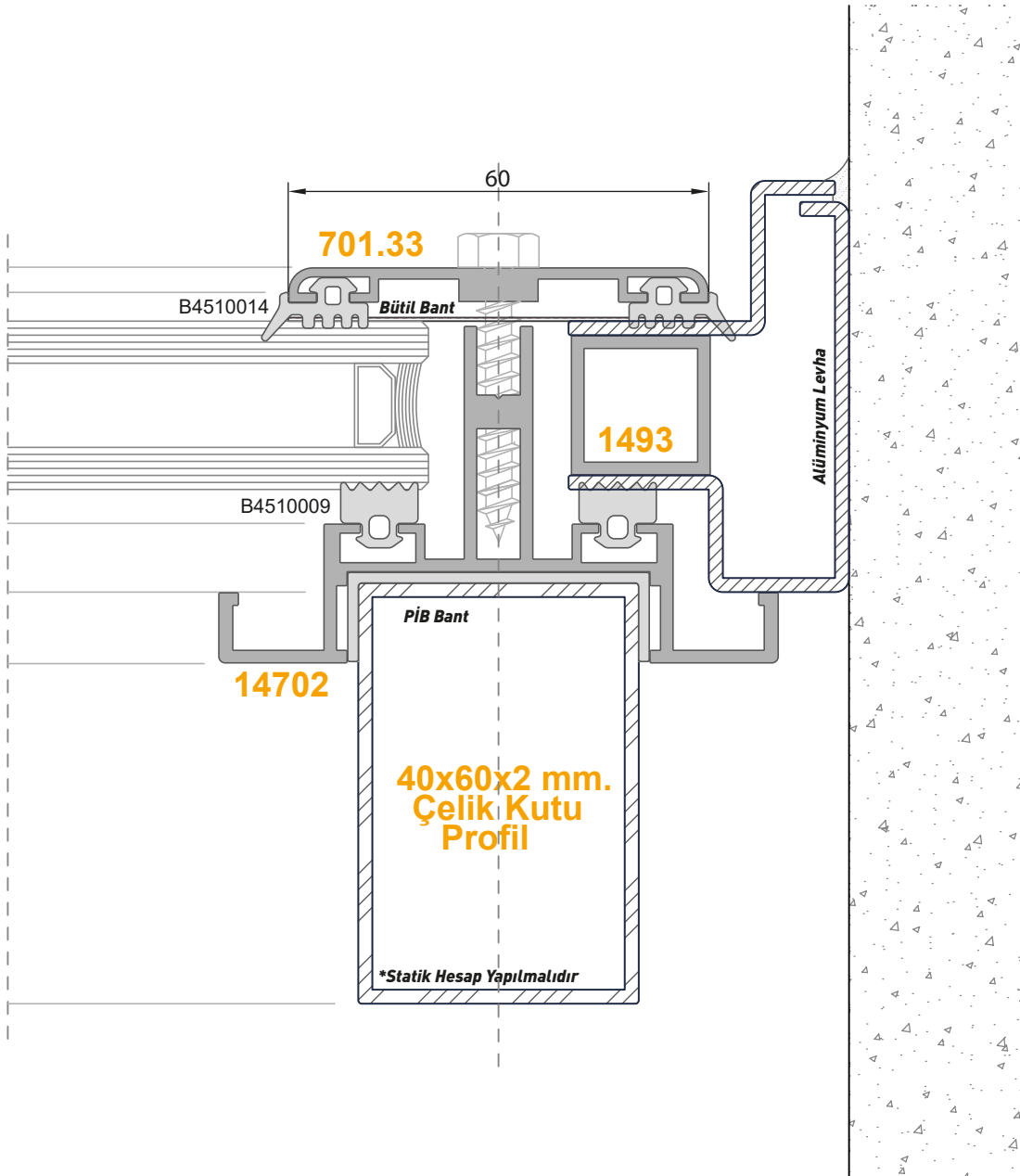
4-4 Detay
