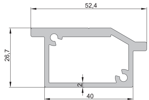
1015 Kanat Profili Sash Profile Ağırlık (Kg/mt.) Weight (Kg/mt.) 1,019 Kg/mt.
