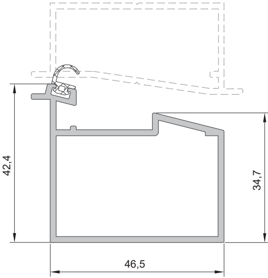
1050 Cam Kapı Kasa Profili Glass Door Case Profile Ağırlık (Kg/mt.) Weight (Kg/mt.) 0,781 Kg/mt.
