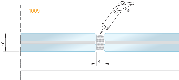
3:3 DETAY 3:3 DETAIL
